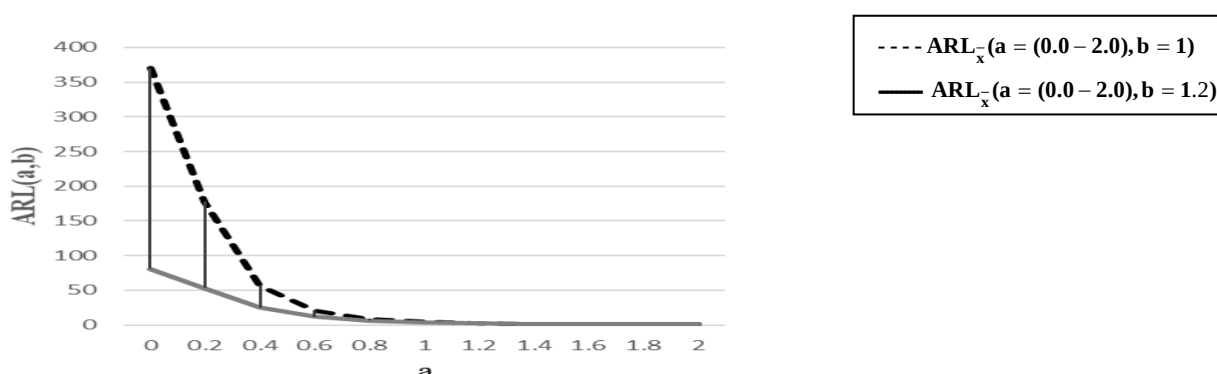
الشكل 4.2 يبين رسم قيم معدلات اطوال التشغيل ARL_{\bar{x}}(a = (0.0 - 2.0), b = 1, 1.2)
