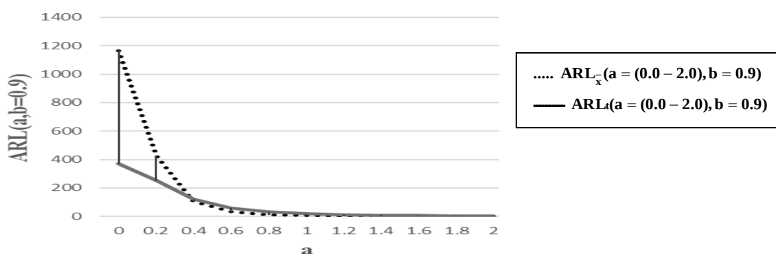
الشكل 5.1. يبين رسم قيم معدلات اطوال التشغيل ARL_{\bar{x}}(a = (0.0 - 2.0), b = 0.9) للوحات سيطرة \bar{X} و ARL_t(a = (0.0 - 2.0), b = 0.9) للوحات سيطرة t - لمتغير المادة الحامضية (x) لمنتج كريم اليد بلسم.
