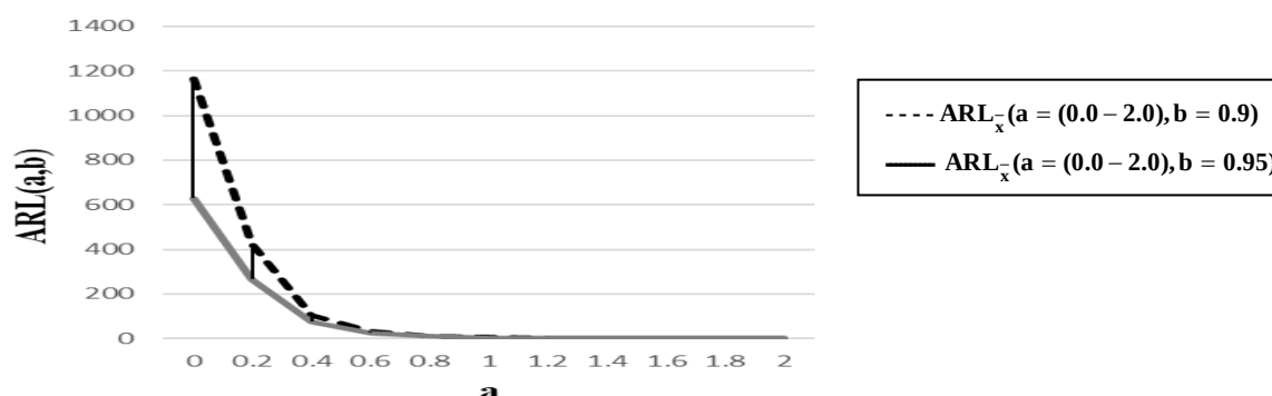
الشكل 4.1 يبين رسم قيم معدلات اطوال التشغيل ARL_{\bar{x}}(a = (0.0 - 2.0), b = 0.9, 0.95)
